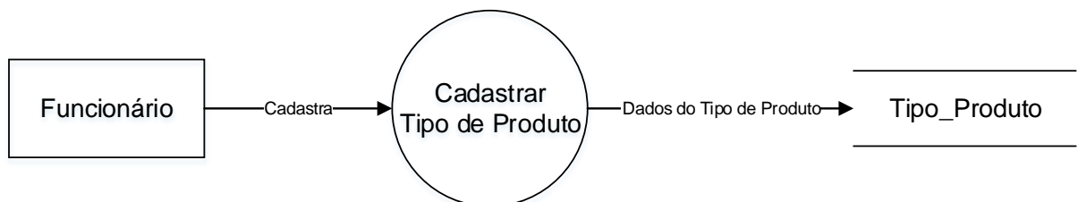
Figura 10 - DFD Tipo de Produto
