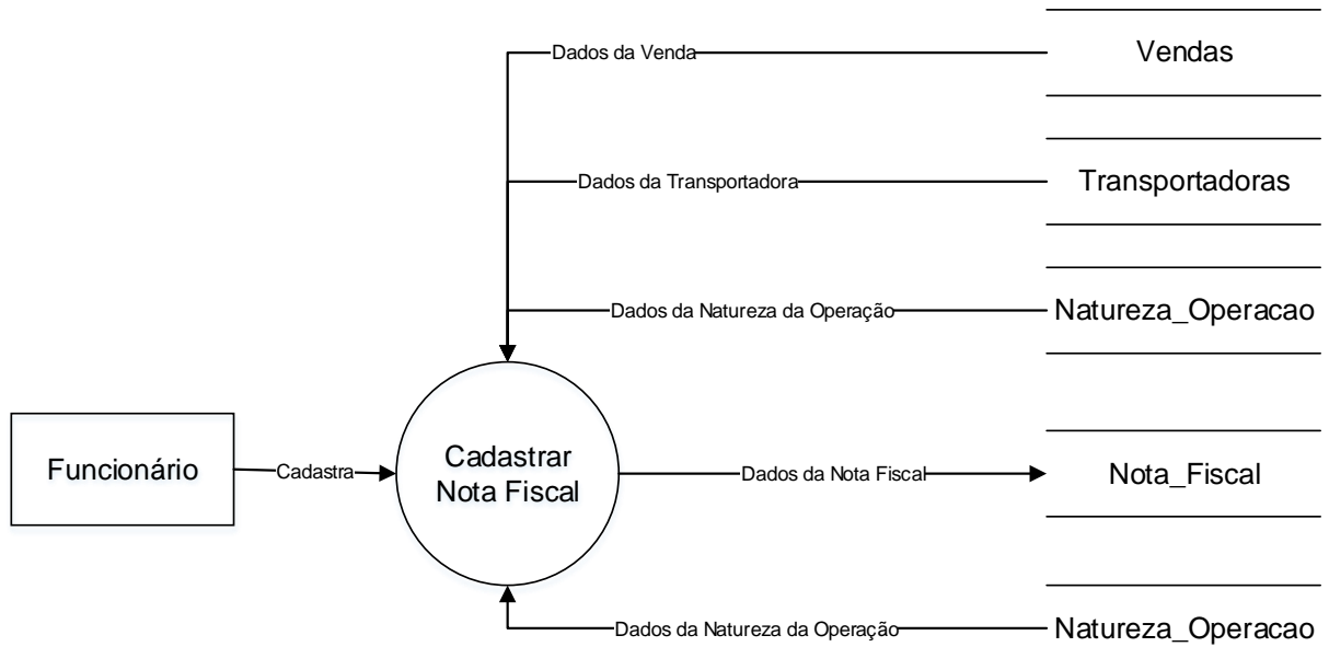
Figura 18 - DFD Nota Fiscal
