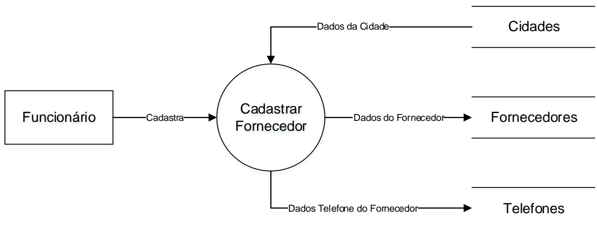
Figura 15 - DFD Fornecedores
