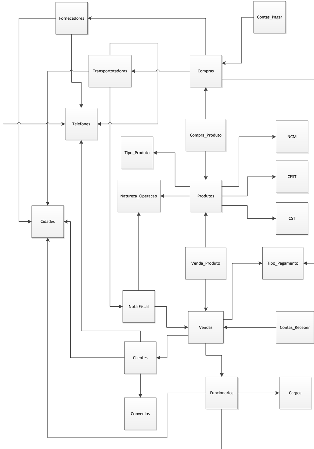
Figura 1 - MER
