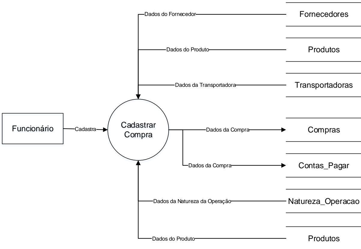
Figura 17 - DFD Compras
