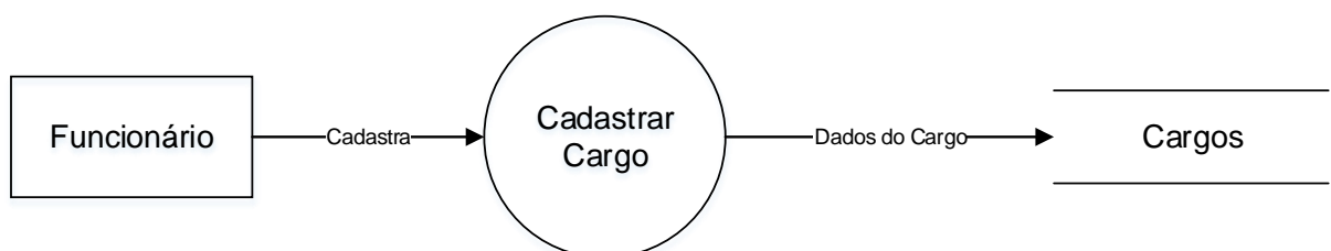
Figura 4 - DFD Cargos
