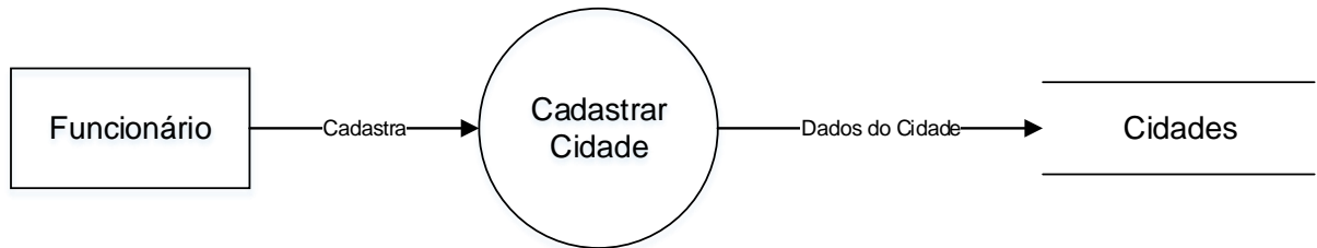
Figura 2 - DFD Cidades
