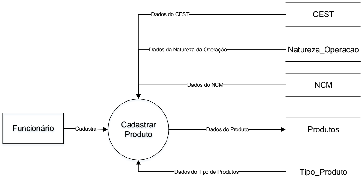
Figura 11 - DFD Produtos
