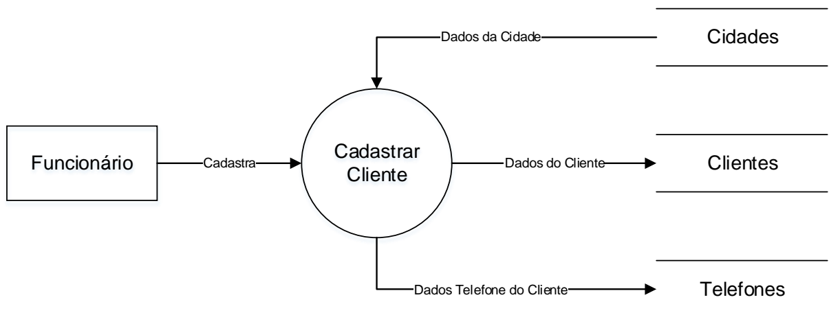
Figura 3 - DFD Clientes
