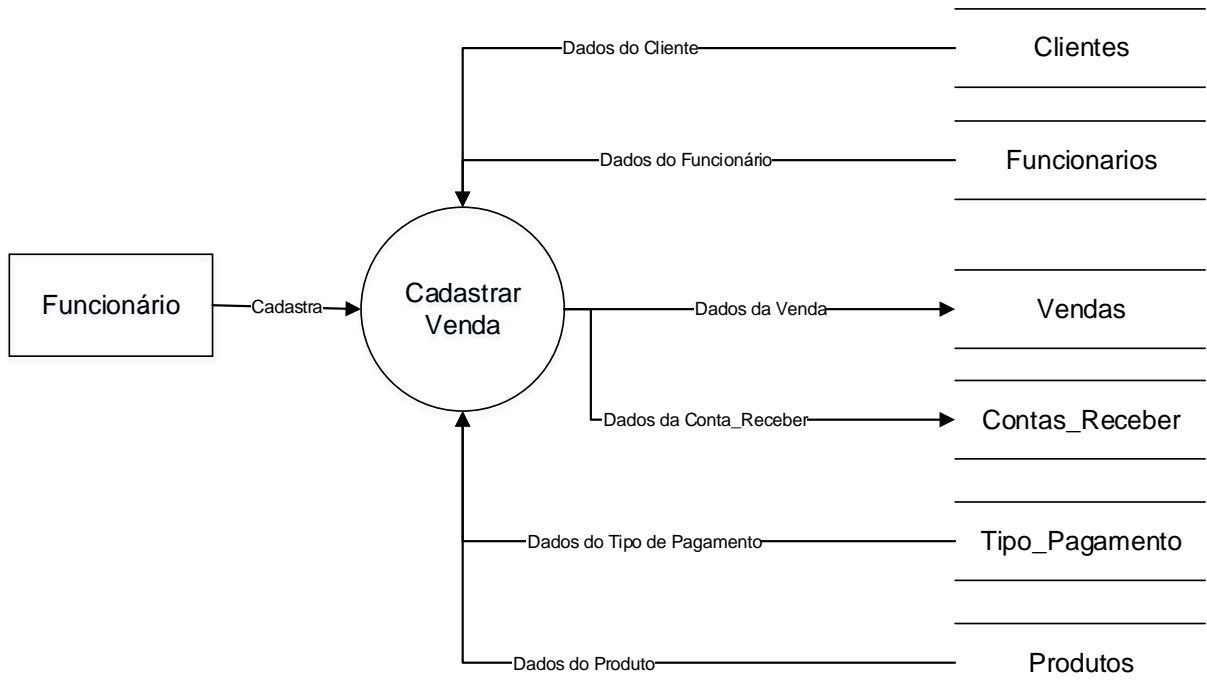
Figura 14 - DFD Vendas
