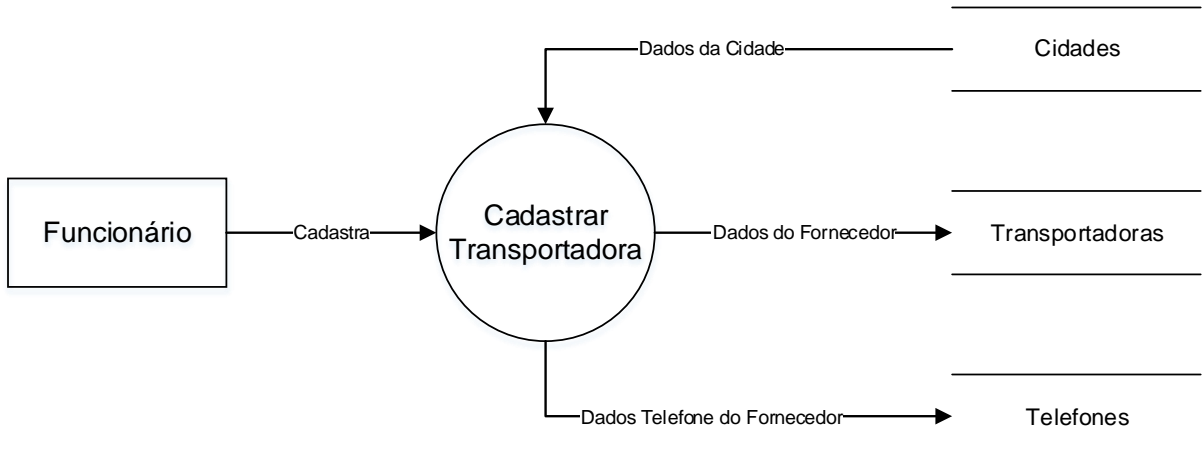
Figura 16 - DFD Transportadoras
