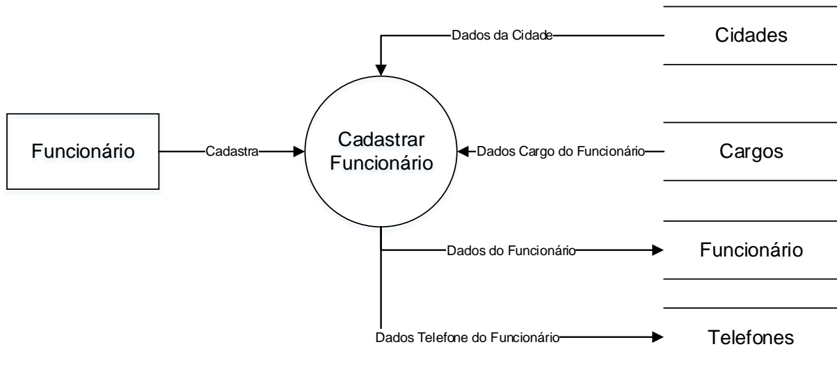
Figura 5 - DFD Funcionários
