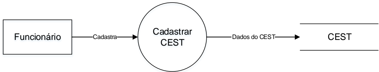
Figura 8 - DFD CEST
