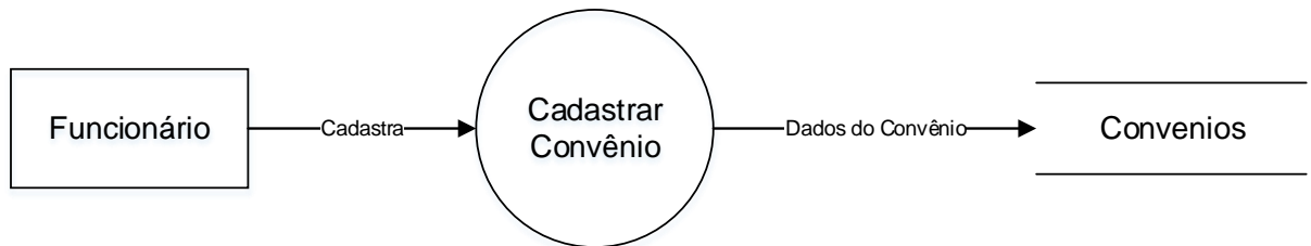
Figura 12 - DFD Convênios
