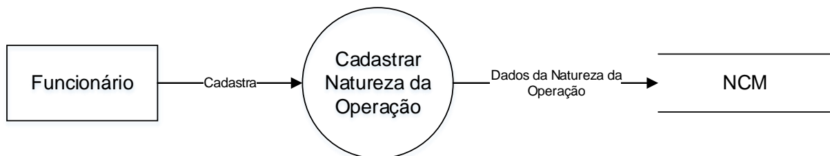
Figura 6 - DFD Natureza da Operação
