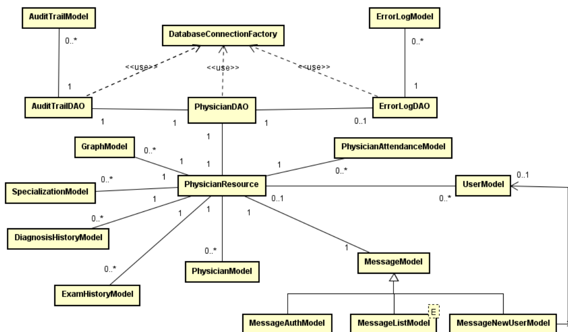
Figura 12 - Diagrama de classe da API de médico (a)
