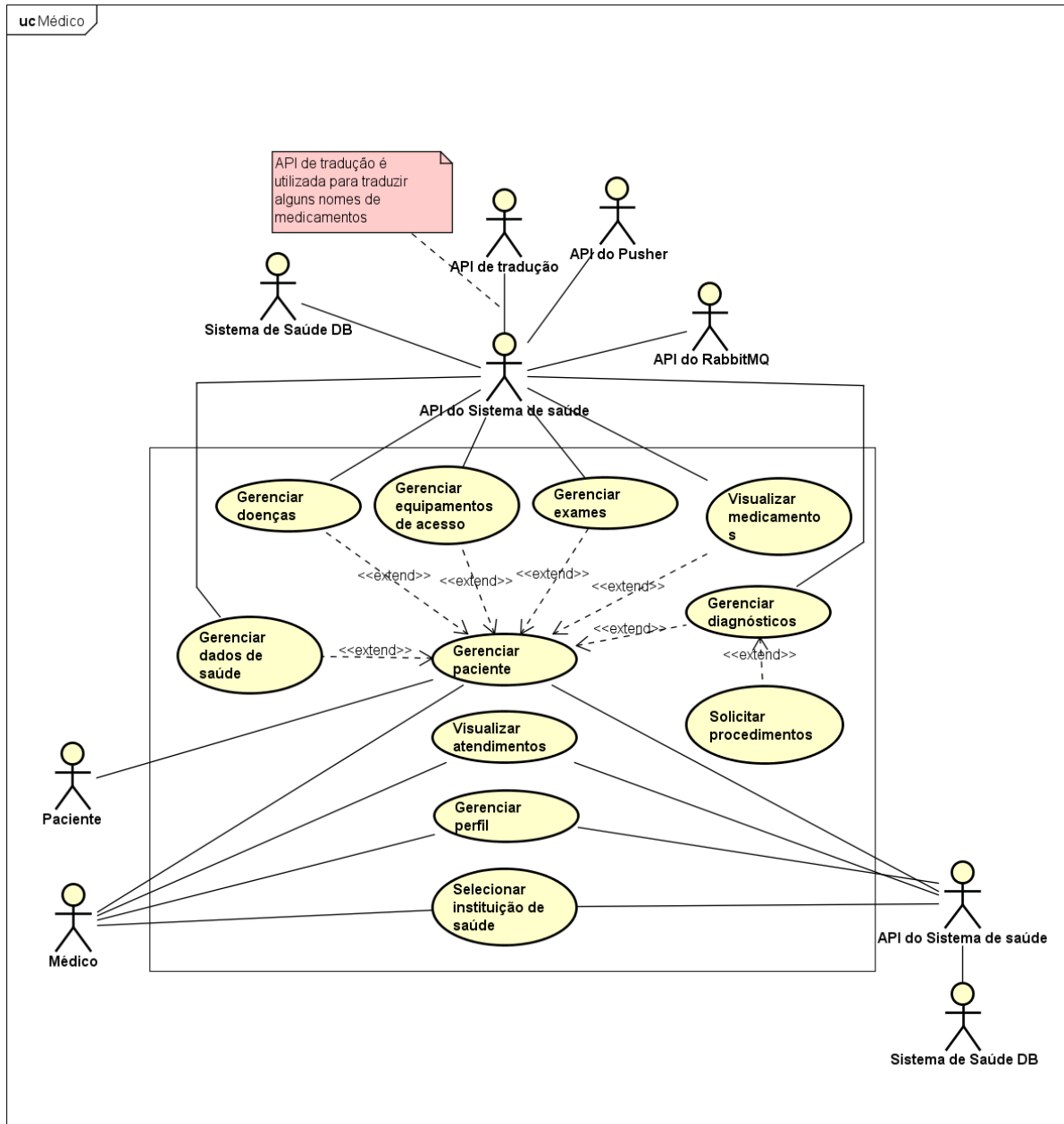
Figura 7 - Diagrama do caso de uso do médico
