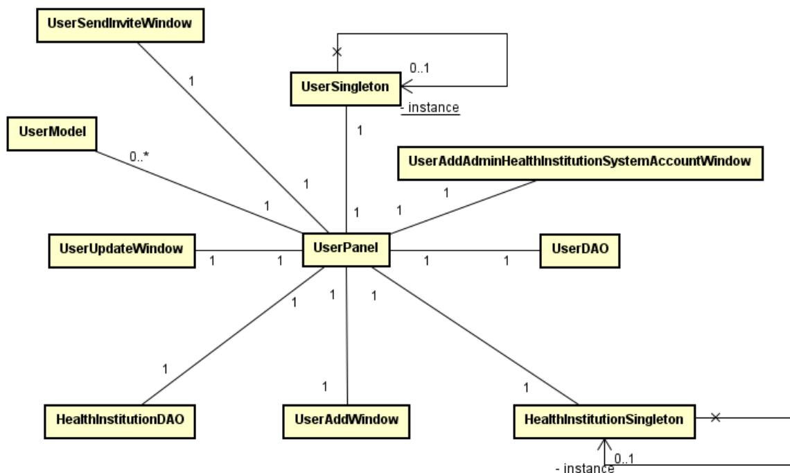
Figura 25 - Diagrama de classe de gerenciar usuários
