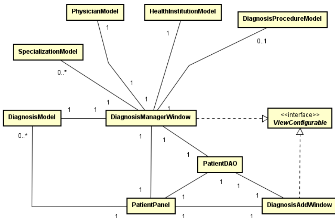
Figura 31 - Diagrama de classe de gestão de diagnósticos do paciente
