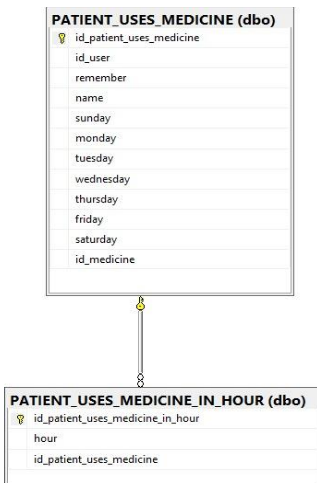
Figura 49 - DER do banco de dados local no dispositivo móvel
