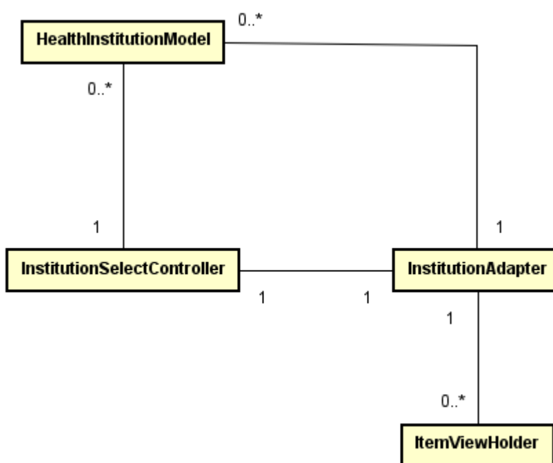
Figura 36 - Diagrama de classe de seleção de instituição de saúde
