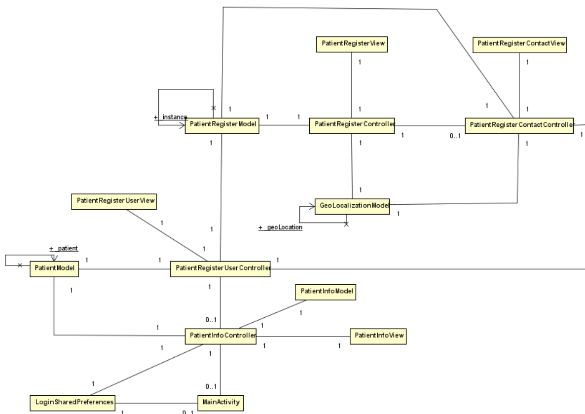
Figura 40 - Diagrama de classe de cadastro de paciente
