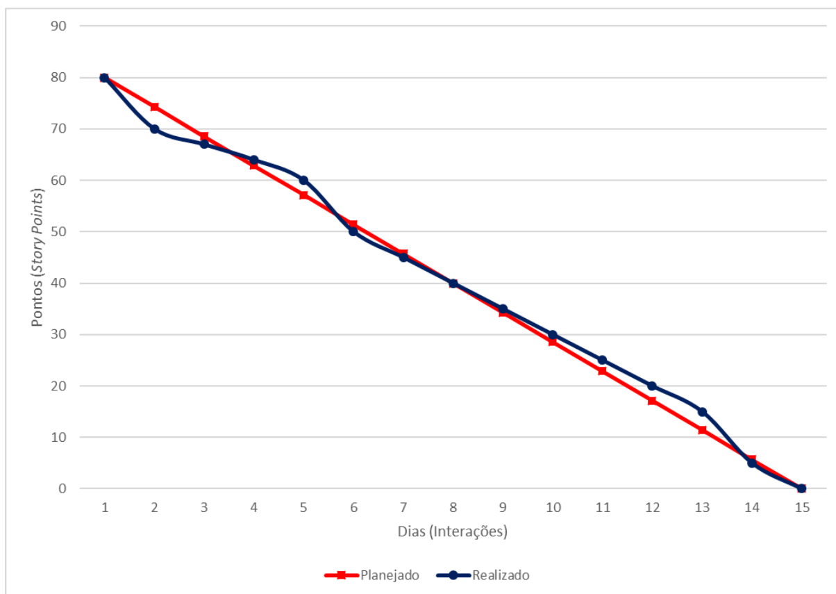
Figura 55 – Gráfico de Burndown da entrega 3.
