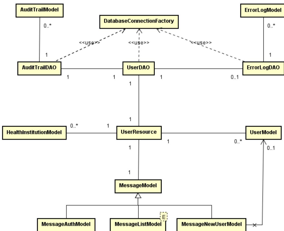
Figura 9 - Diagrama de classe da API de Usuários
