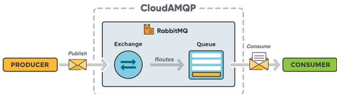
Figura 1 - CloudAMQ e RabbitMQ
