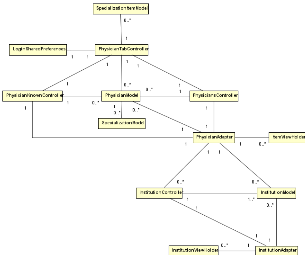
Figura 43 - Diagrama de classe de listagem de médicos(as)
