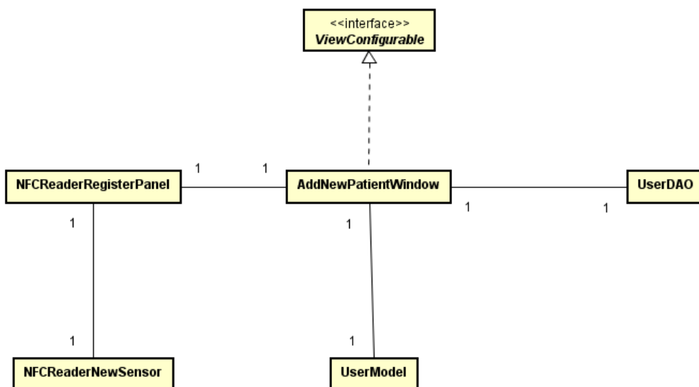
Figura 29 - Diagrama de classe de adicionar novo paciente
