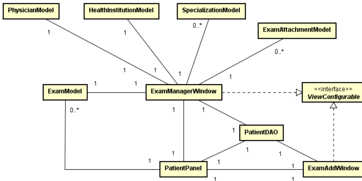
Figura 32 - Diagrama de classe de gerenciamento de exames
