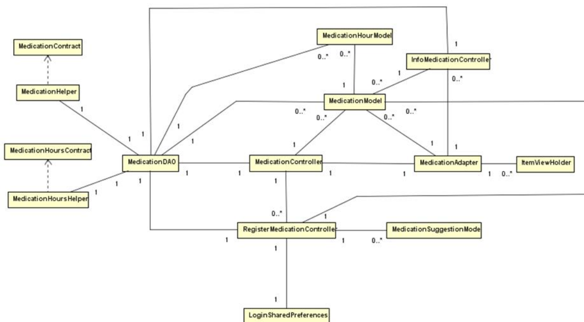
Figura 44 - Diagrama de classe de gerenciamento de medicamentos
