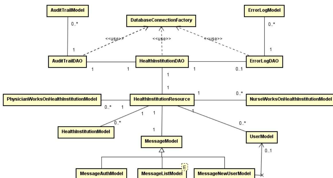
Figura 14 - Diagrama de Classe da API de instituição de saúde
