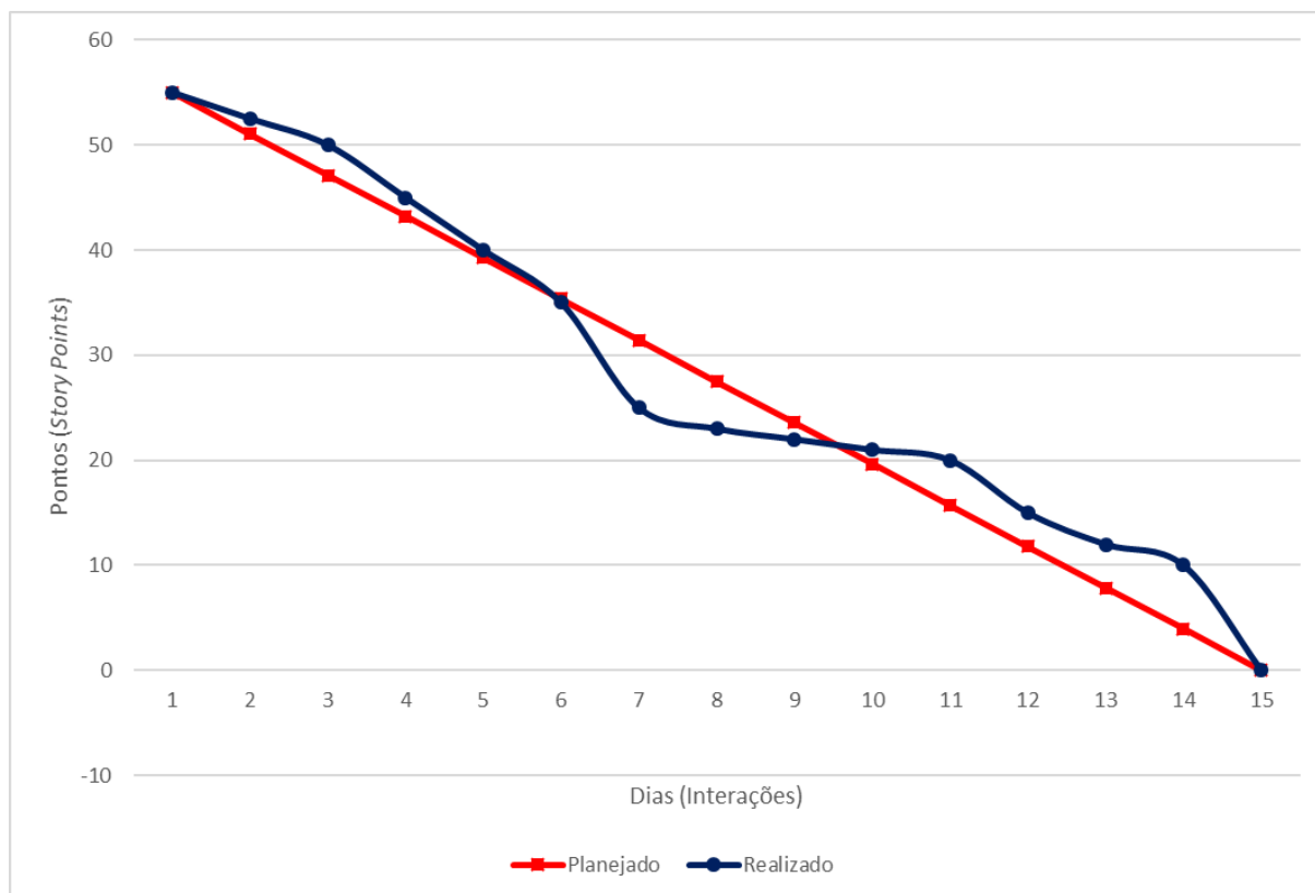
Figura 57 – Gráfico de Burndown da entrega 5.
