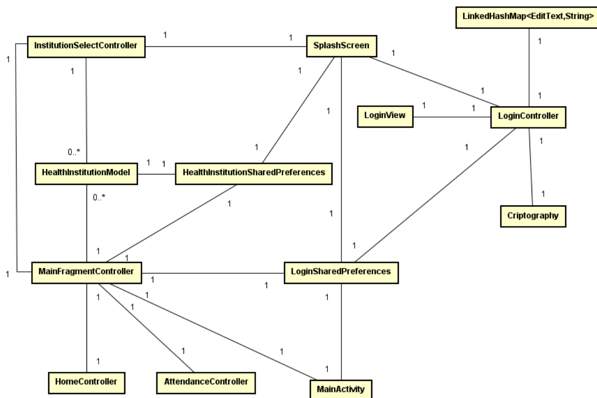
Figura 35 - Diagrama de classe de Login e Navegação
