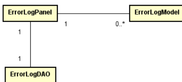
Figura 22 - Diagrama de classe de log de erros
