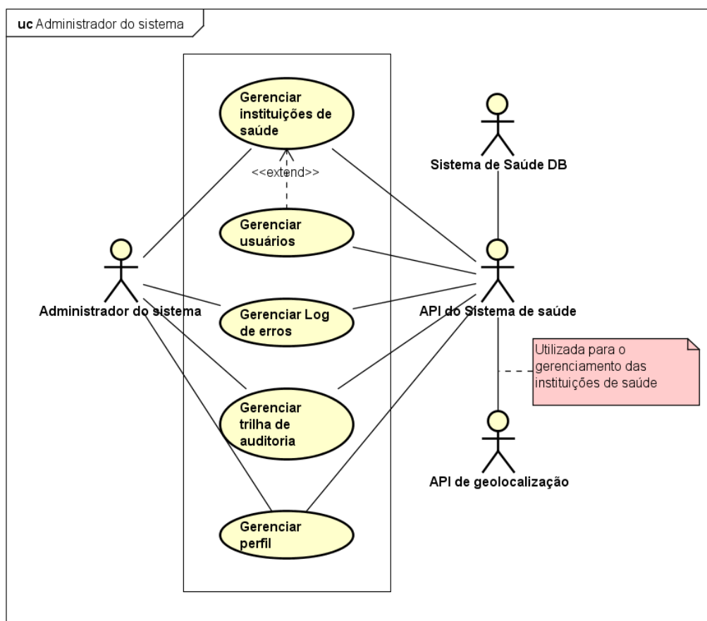
Figura 4 - Diagrama de caso de uso do administrador do sistema
