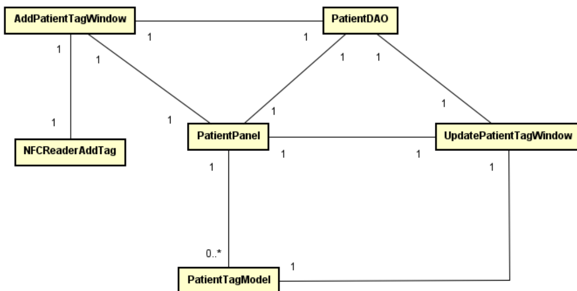
Figura 34 - Diagrama de classe de gerenciar equipamentos de acesso
