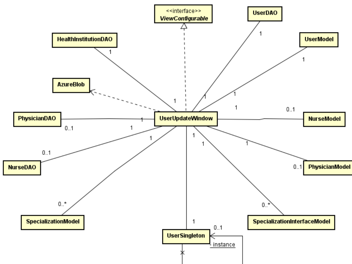
Figura 23 - Diagrama de classe de alterar perfil
