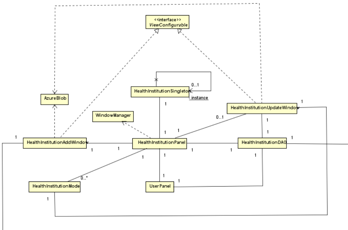
Figura 19 - Diagrama de classe do gerenciamento de instituições de saúde
