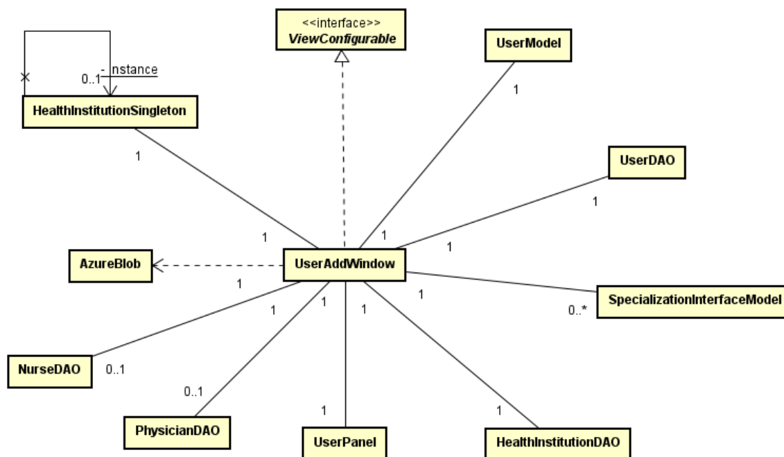
Figura 26 – Diagrama de classe de adicionar usuário na instituição de saúde
