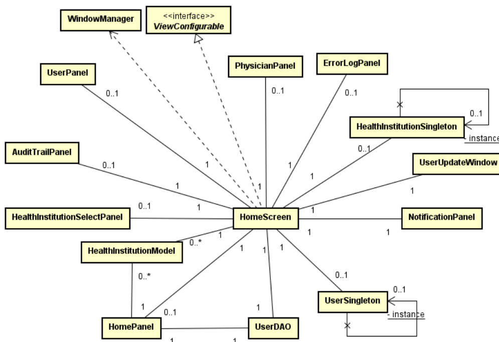
Figura 18 - Diagrama de classe da navegação do sistema
