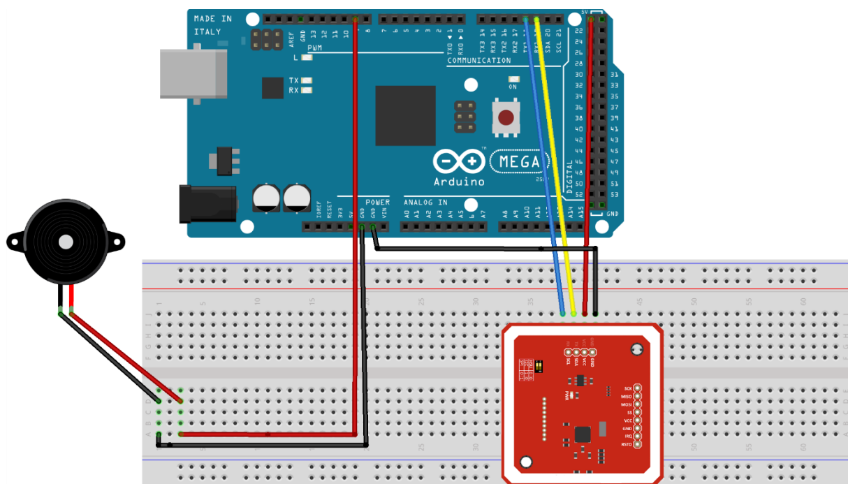
Figura 50 - Circuito
