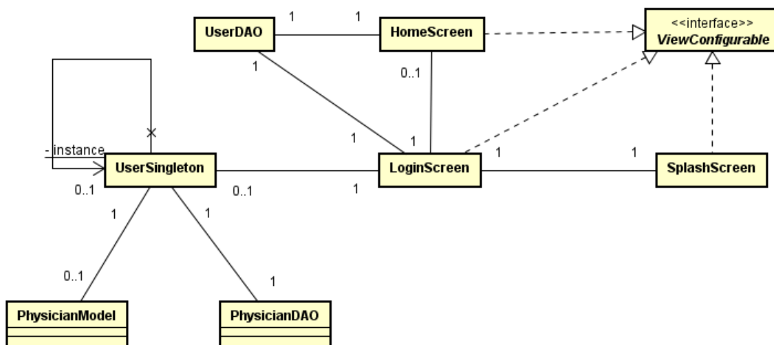
Figura 17 - Diagrama de classe da funcionalidade de Login
