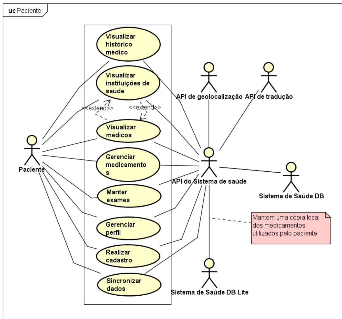
Figura 8 - Diagrama de caso de uso paciente
