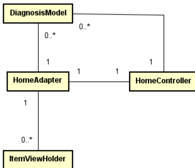
Figura 37 - Diagrama de classe de listagem de novos pacientes na fila
