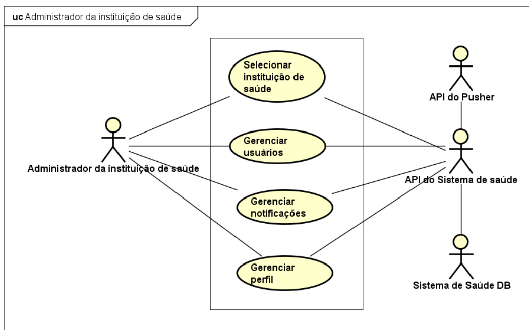
Figura 5 - Diagrama de caso de uso do administrador da instituição de saúde
