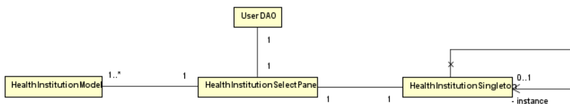
Figura 20 - Diagrama de classe da seleção de instituição de saúde
