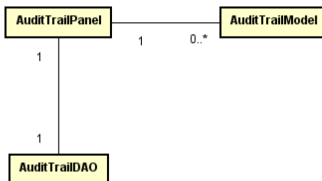
Figura 21 - Diagrama de classe da trilha de auditoria
