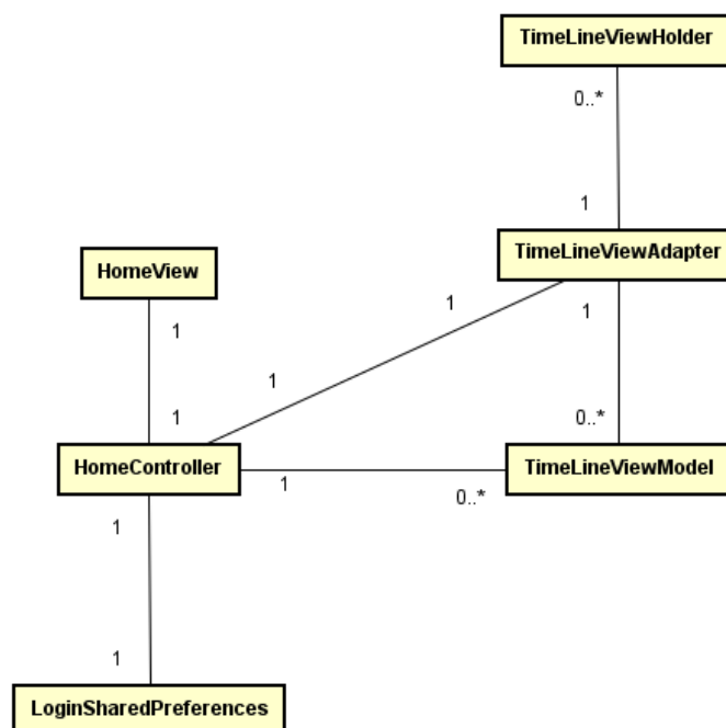
Figura 41 - Diagrama de classe da tela inicial do sistema
