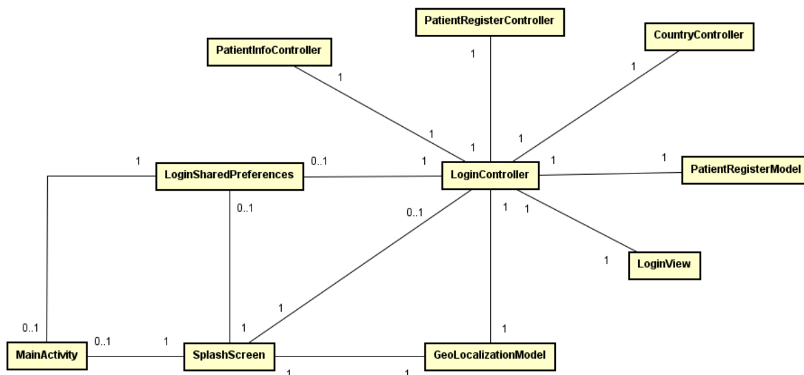
Figura 39 - Diagrama de classe da funcionalidade de inicialização
