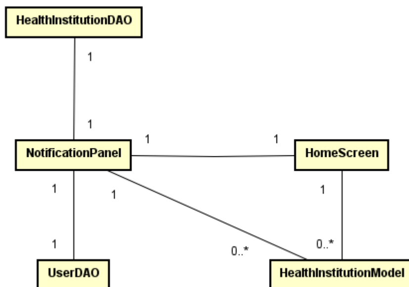
Figura 24 - Diagrama de classe de notificação
