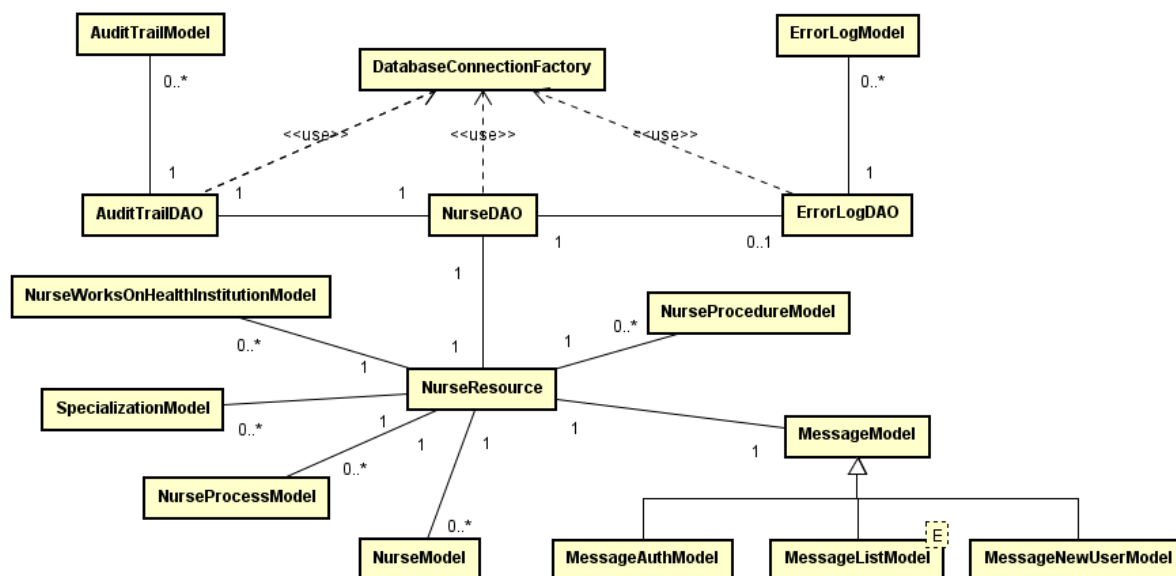
Figura 13 - Diagrama de Classe da API da Enfermeira
