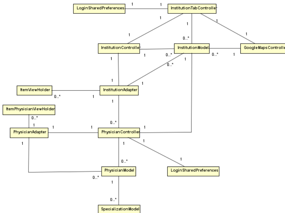
Figura 42 - Diagrama de classe de listagem de instituições de saúde próximas
