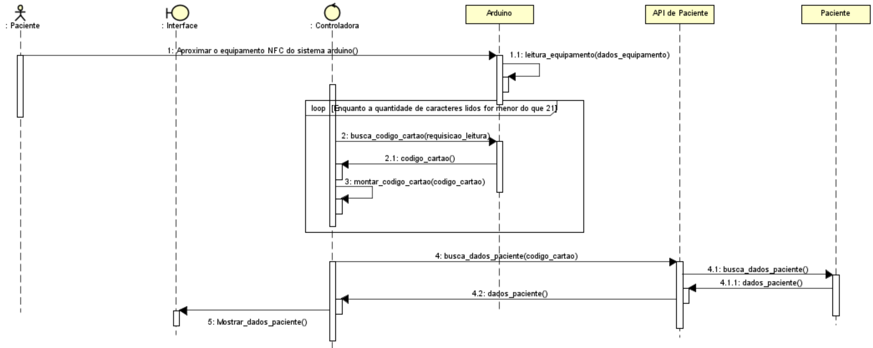
Figura 47 - Diagrama de sequência da leitura do equipamento NFC
