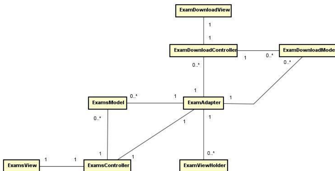
Figura 46 - Diagrama de classe de exames
