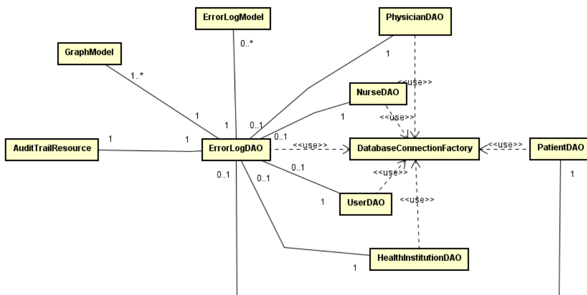
Figura 16 - Diagrama de Classe da API de Erro
