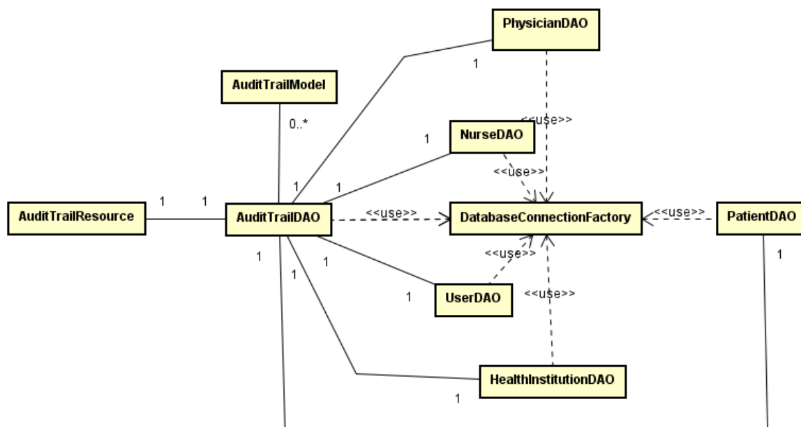
Figura 15 - Diagrama de Classe da API de trilha de auditoria
