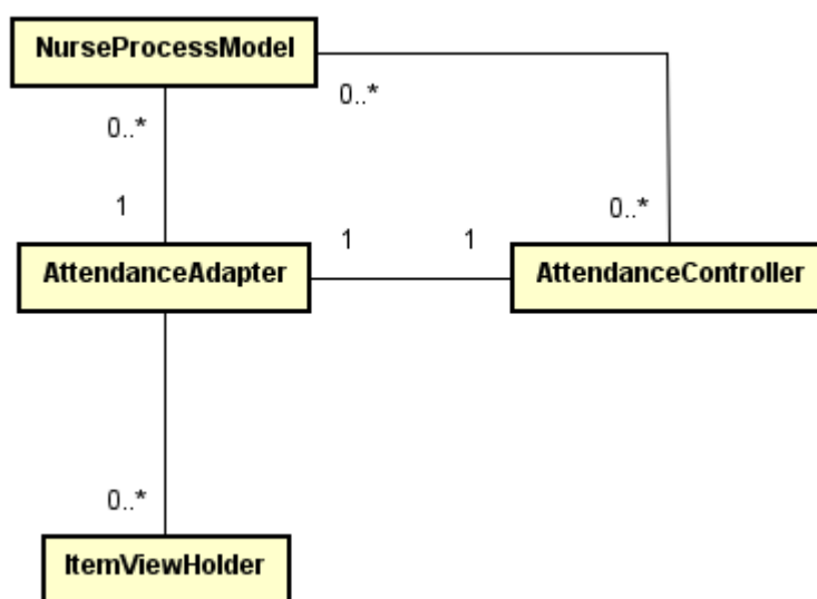
Figura 38 - Diagrama de classe de gerenciar lista de atendimentos em progresso
