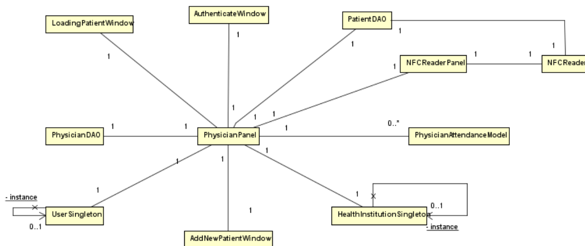
Figura 27 - Diagrama de classe de gerenciamento de pacientes
