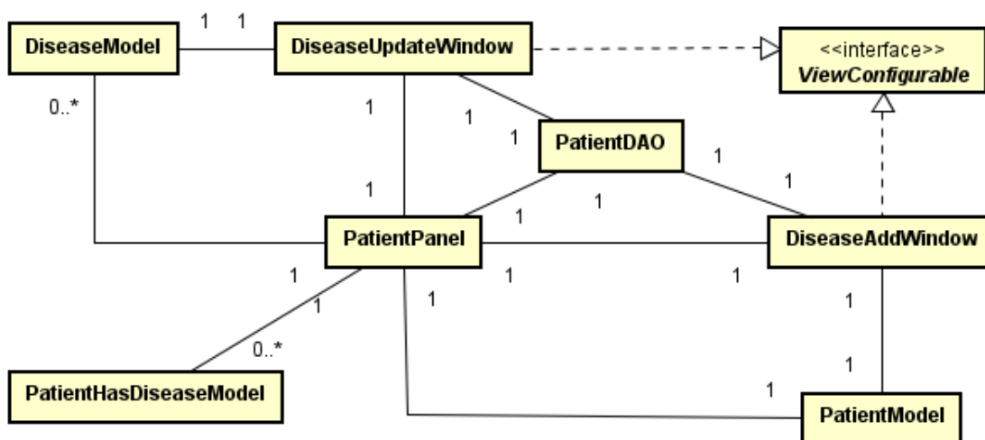
Figura 30 - Diagrama de classe de gerenciamento das doenças do paciente
