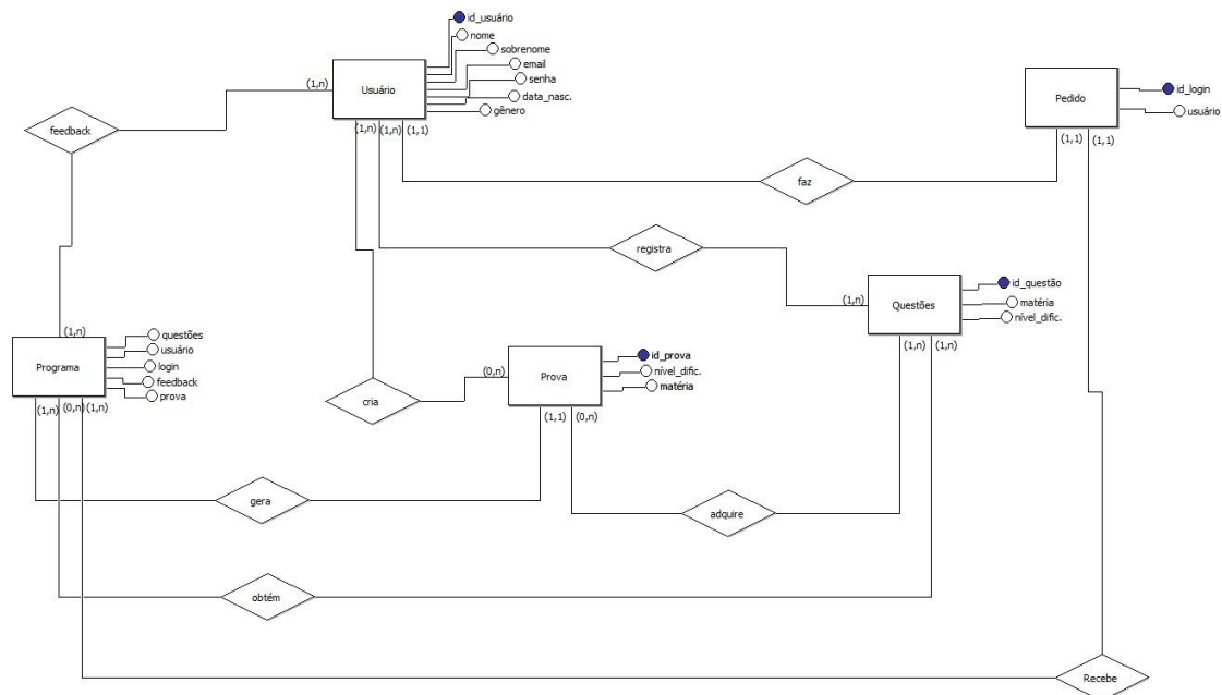
Figura 11 – Modelo Lógico do Banco de Dados
