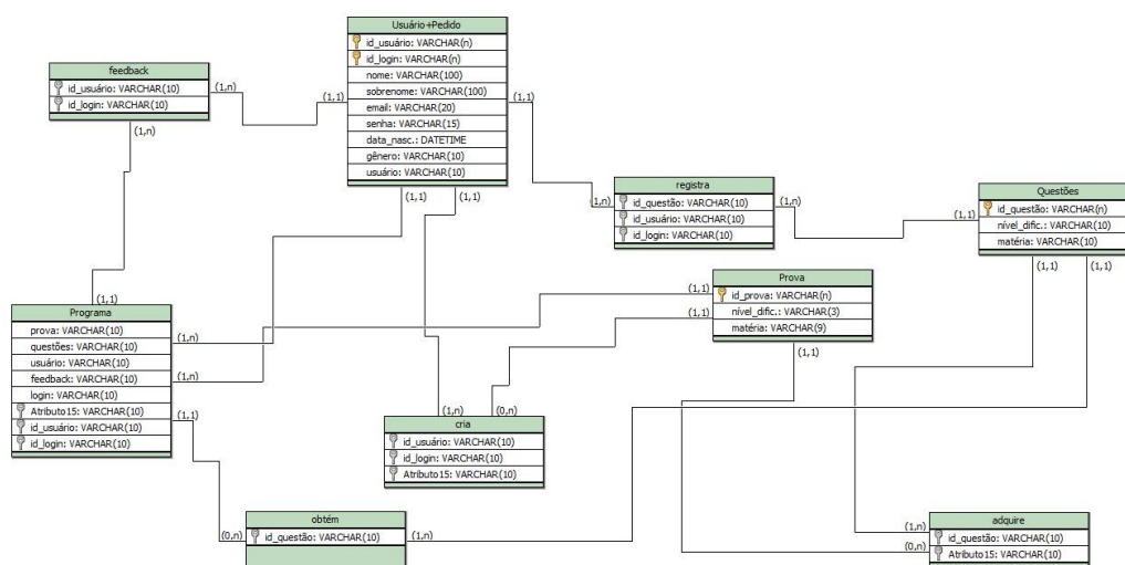
Figura 10 – Modelo Lógico do Banco de Dados
