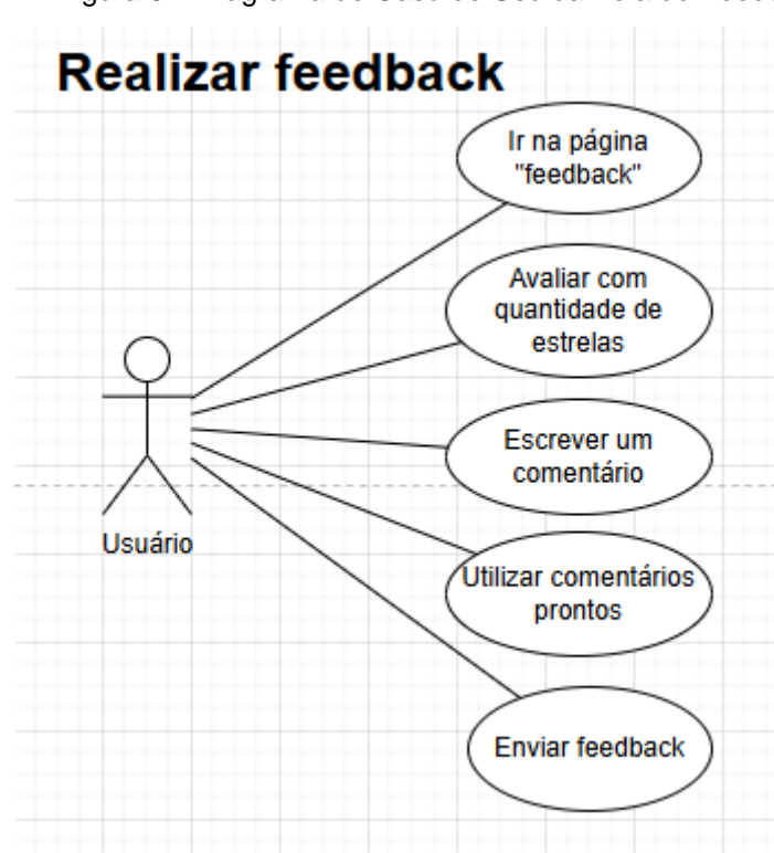
Figura 8 – Diagrama de Caso de Uso da Tela de Feedback
