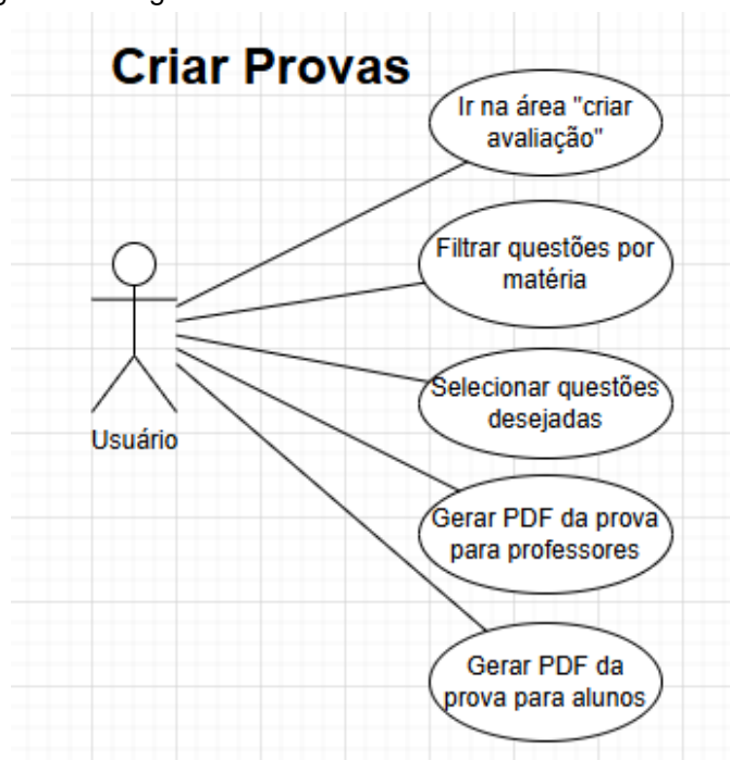
Figura 7 – Diagrama de Caso de Uso da Tela de Criar Avaliações
