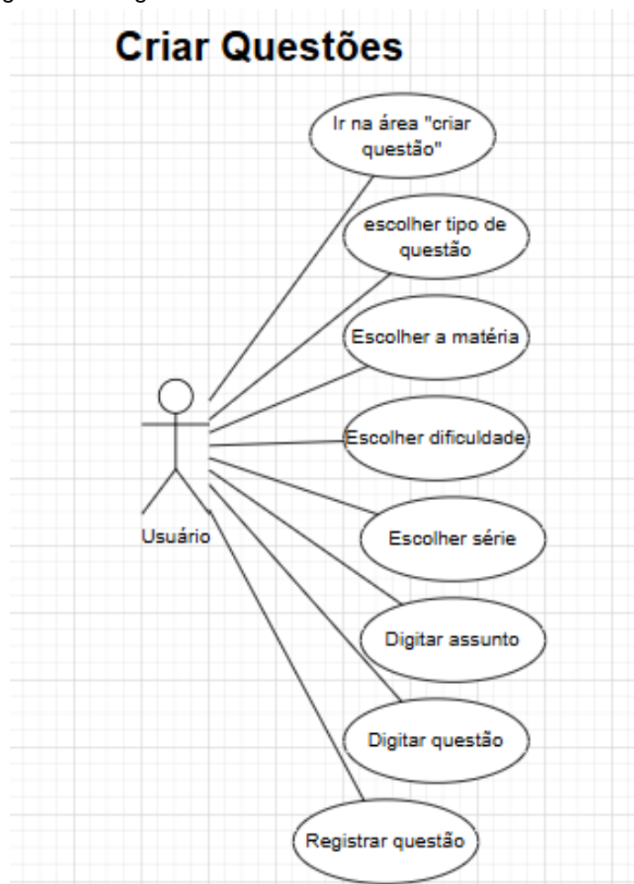
Figura 6 – Diagrama de Caso de Uso da Tela de Criar Questões
