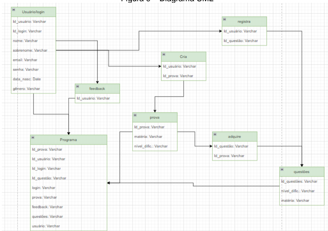
Figura 9 – Diagrama UML
