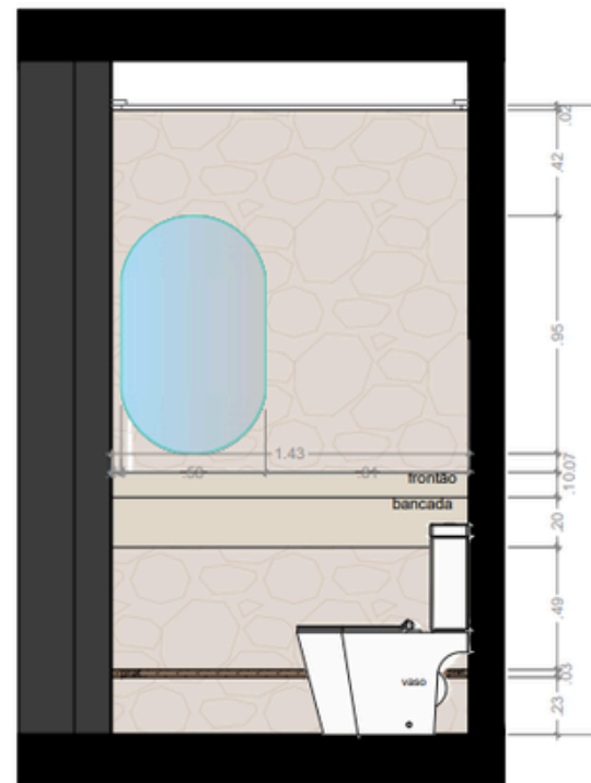
LAVABO VISTA 01
