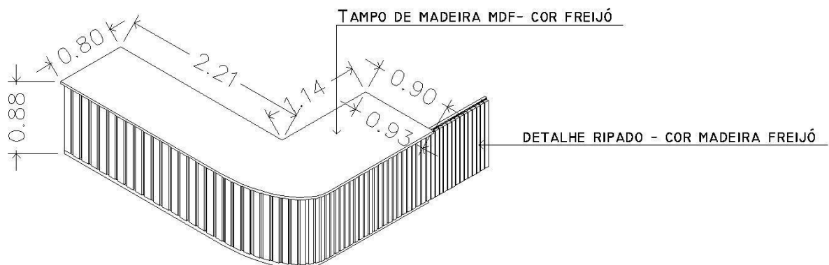
PERSPECTIVA- BALCÃO DE ATENDIMENTO SEM ESCALA
