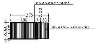
VISTA LAT. ESQ. - BALCÃO DE ATENDIMENTO SEM ESCALA
