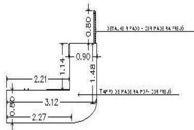
VISTA SUPERIOR - BALCÃO DE ATENDIMENTO SEM ESCALA
