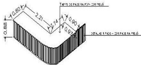
PERSPECTIVA - BALCÃO DE ATENDIMENTO SEM ESCALA
