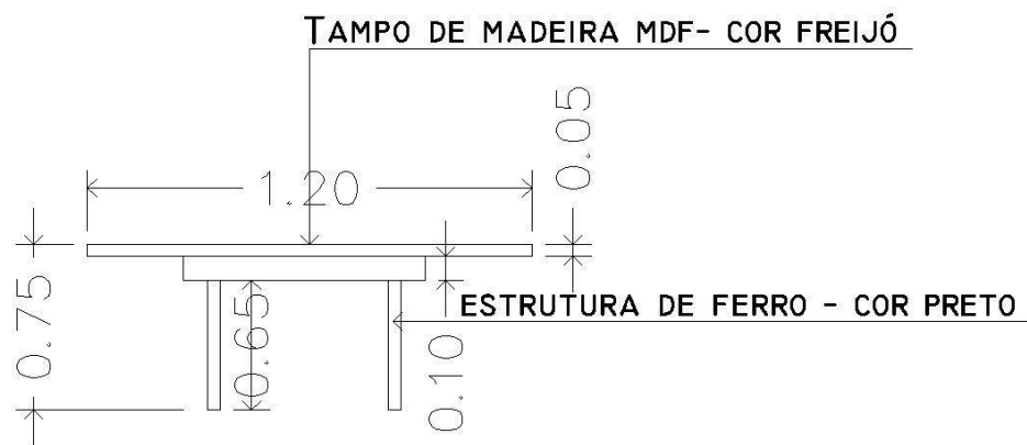
VISTA FRONTAL- MESA ORGÂNICA SEM ESCALA
