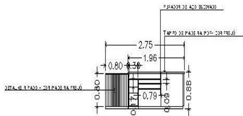
VISTA LAT. DIREITA - BALCÃO DE ATENDIMENTO SEM ESCALA
