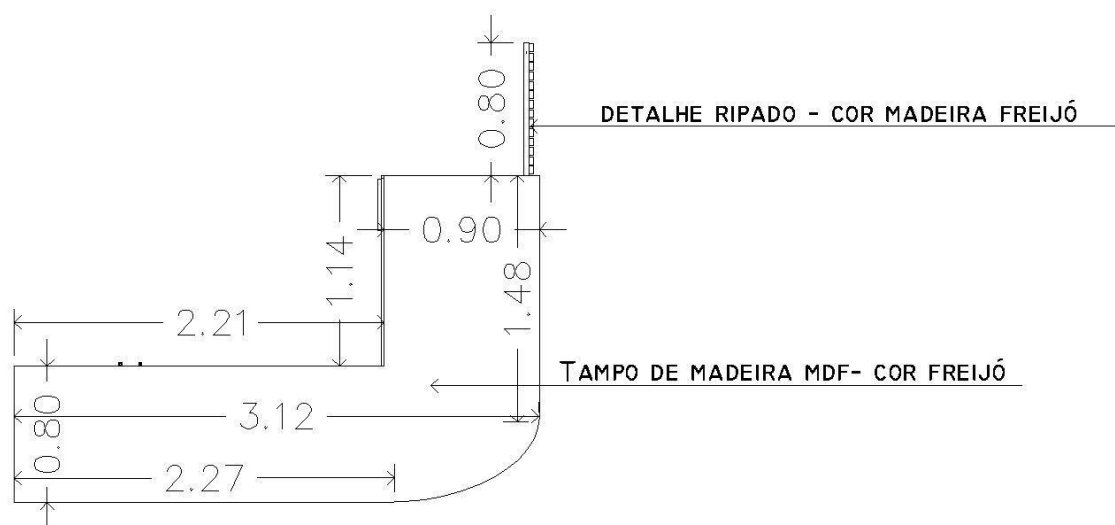
VISTA SUPERIOR - BALCÃO DE ATENDIMENTO SEM ESCALA
