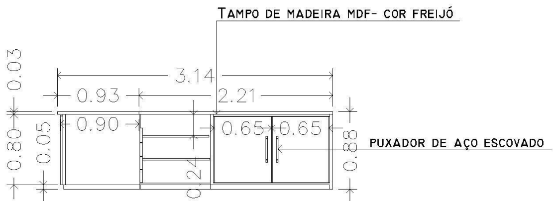
VISTA FRONTAL- BALCÃO DE ATENDIMENTO SEM ESCALA
