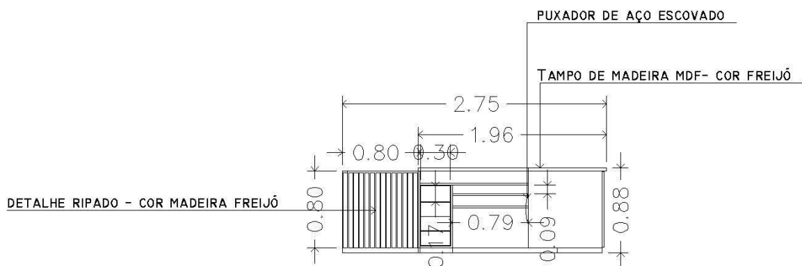
VISTA LAT.DIREITA.- BALCÃO DE ATENDIMENTO SEM ESCALA
