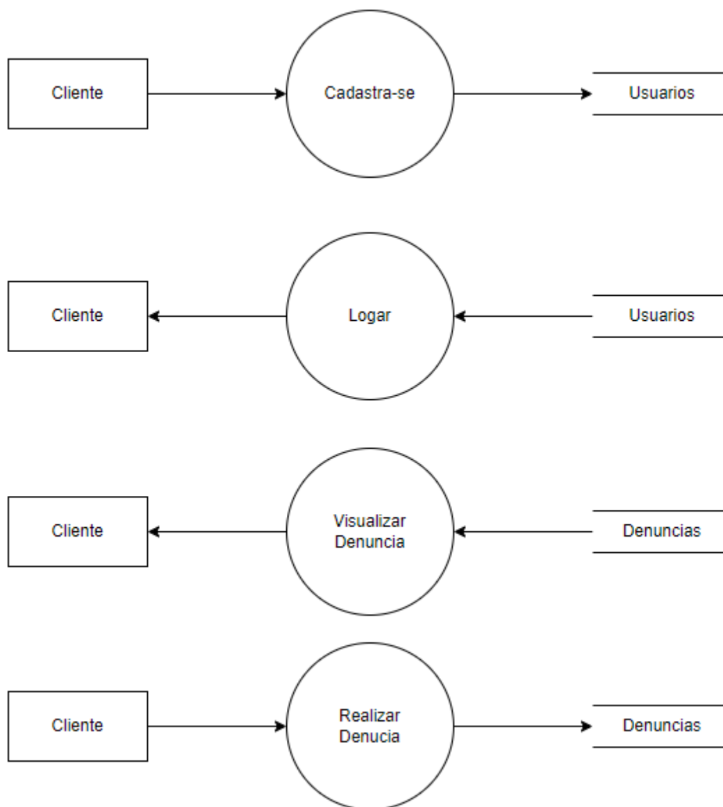
Figura 2 - DFD
