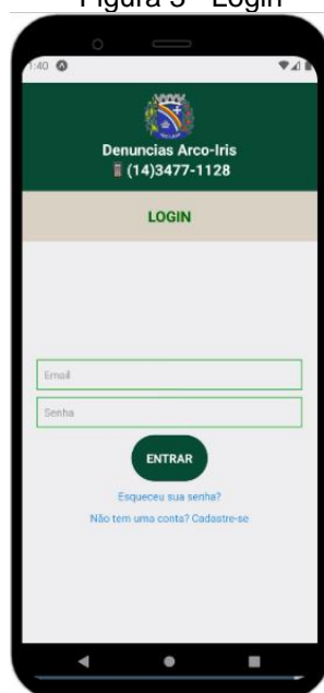
Figura 3 - Login
