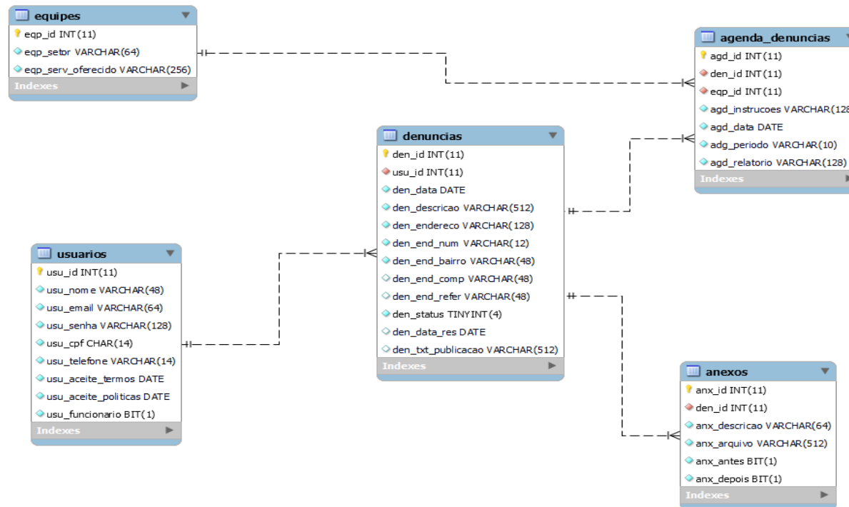
Figura 1 - MER
