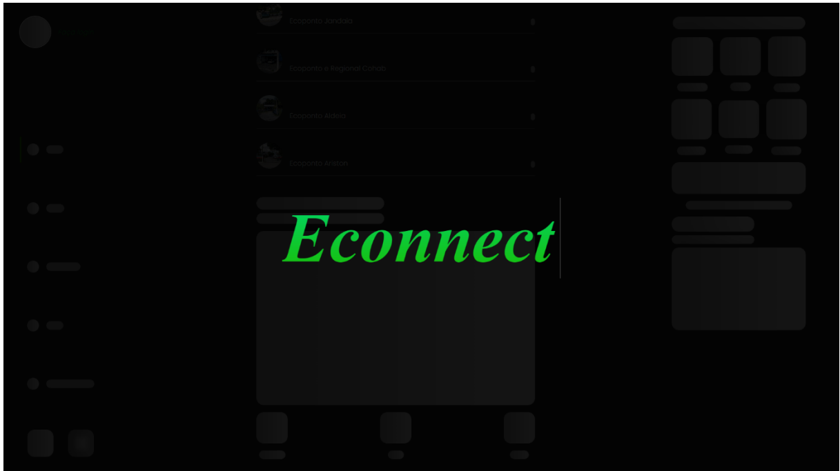
Figura 3 - Pré Loader.
