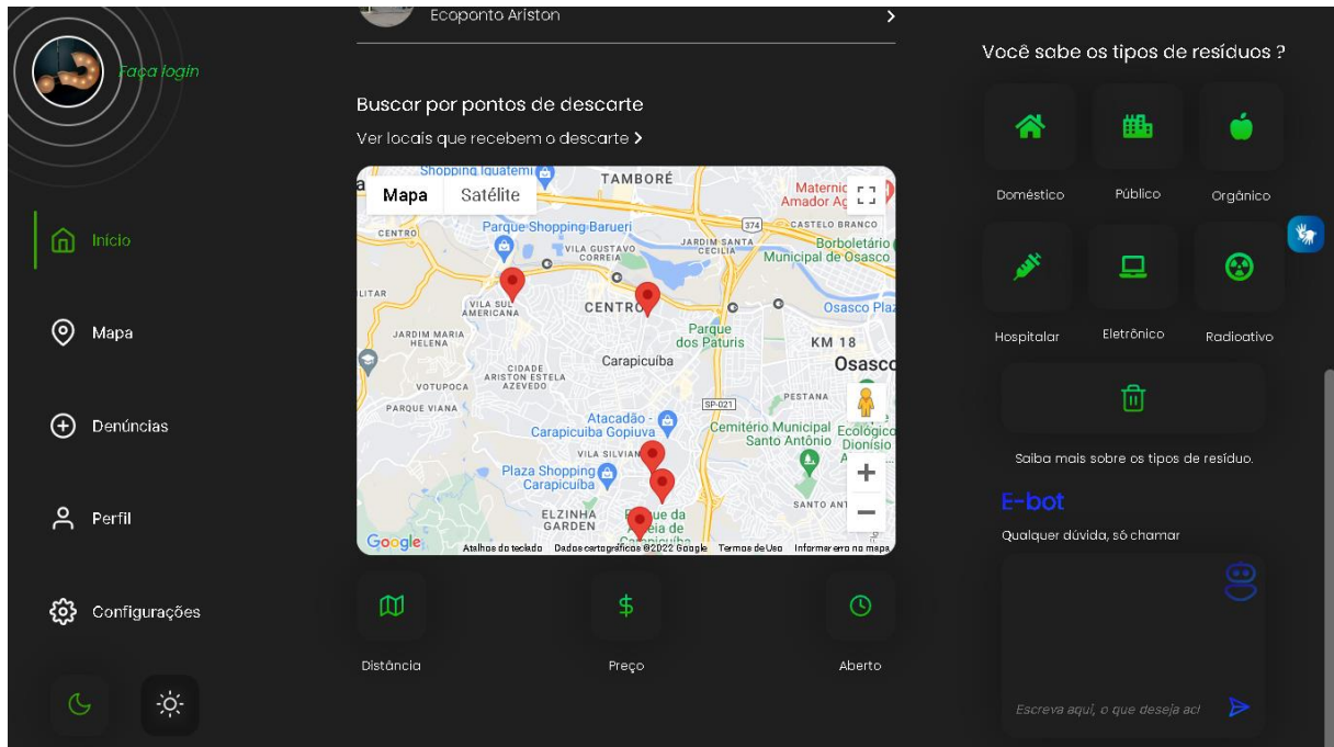
Figura 6 – Página home/início 2.
