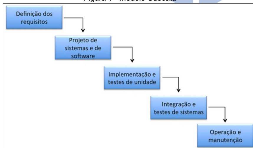
Figura 1 - Modelo Cascata
