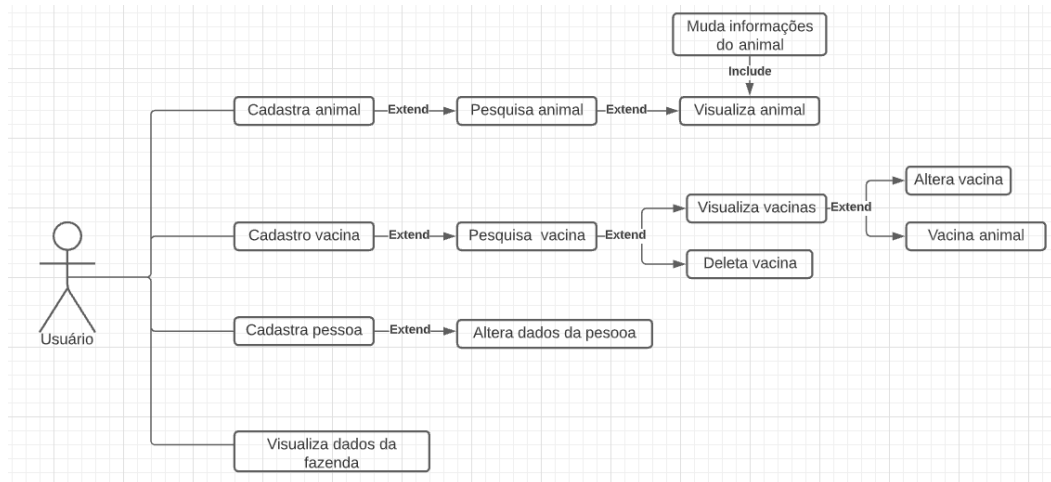
Figura 09 – Diagrama de Caso de Uso
