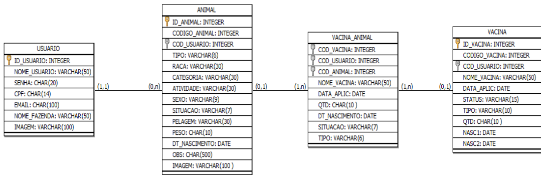
Figura 08 – Banco de Dados
