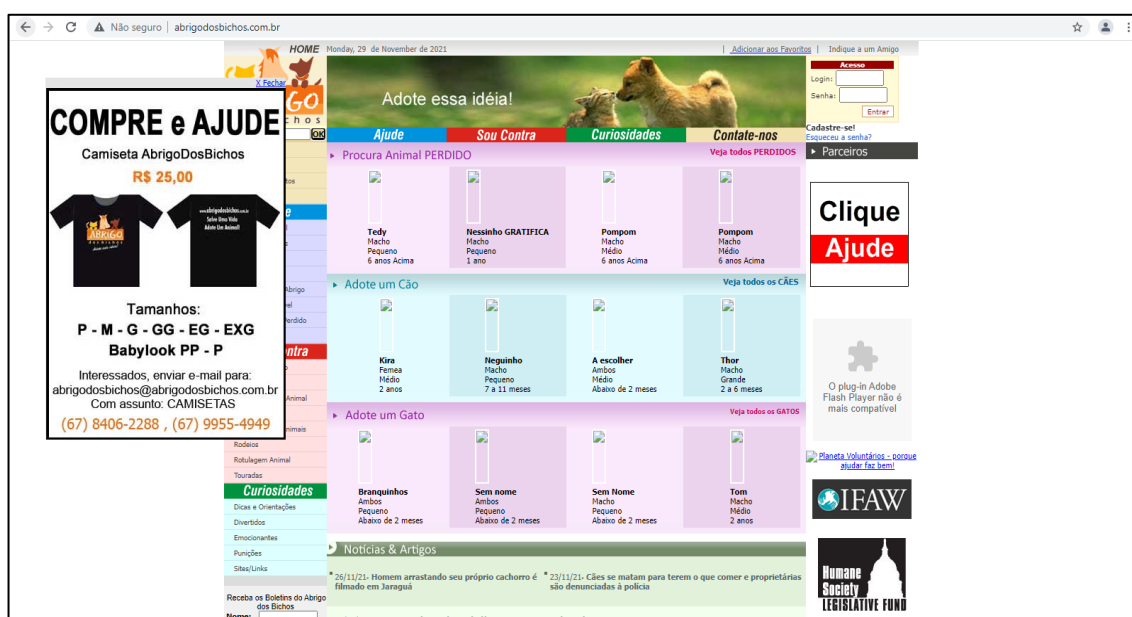
Figura 6– Site Abrigo dos Bichos, tela de adoção.
