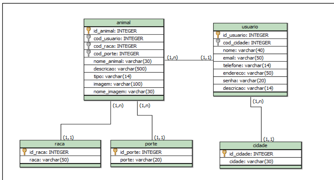
Figura 9– Banco de Dados
